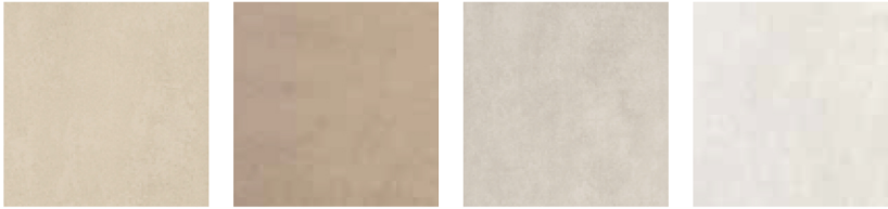
sabbia
